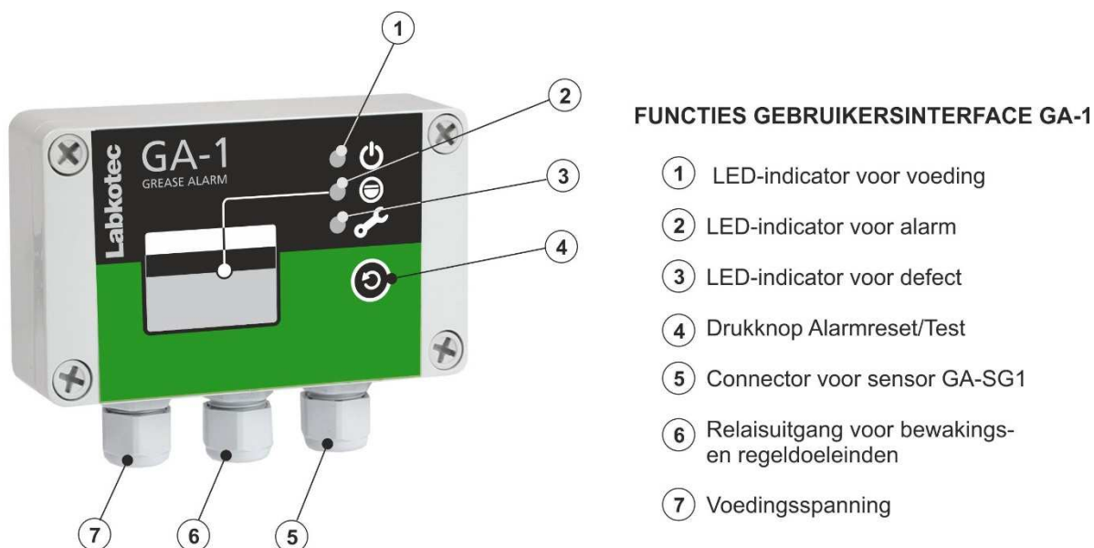
Afbeelding 2. Functies van regeleenheid GA-1
