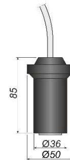
Afbeelding 8. Sensor GA-SG1
