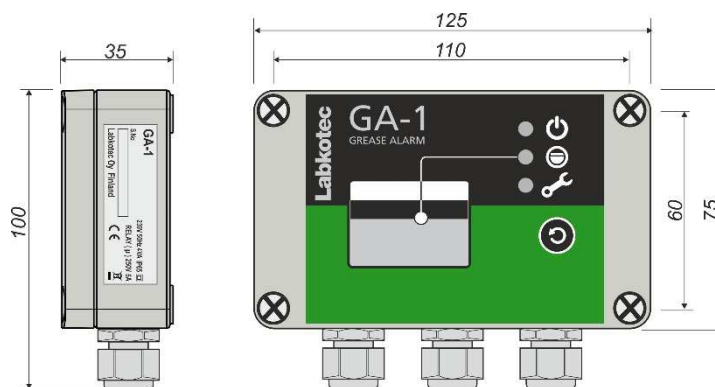
Afbeelding 7. Regeleenheid GA-1
