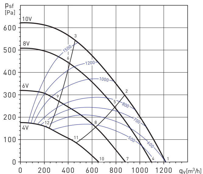
CAB-250 ECOWATT
