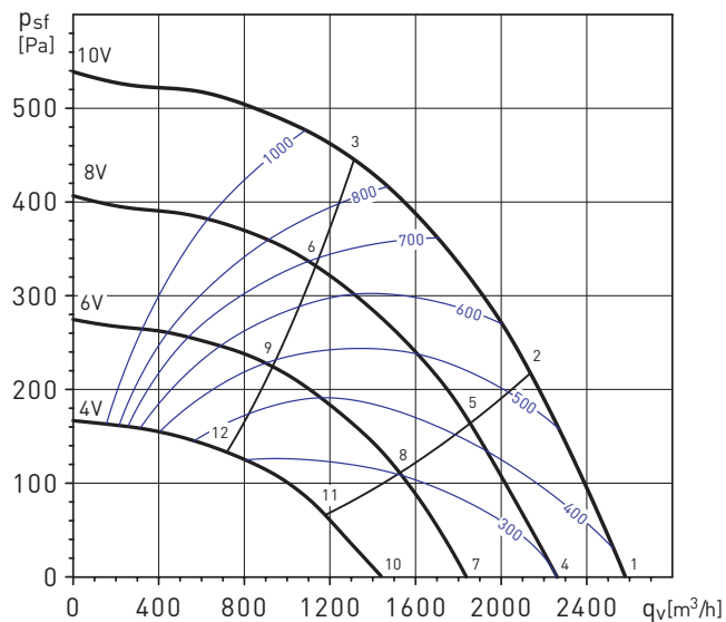
CAB-355 ECOWATT
