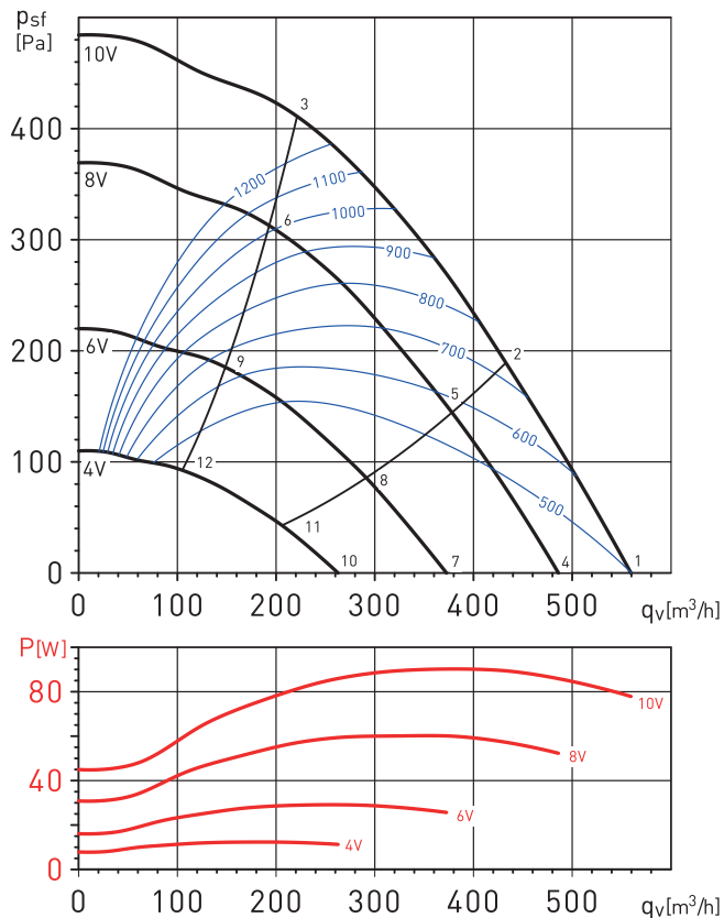
CAB-150 ECOWATT
