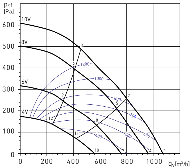
CAB-200 ECOWATT
