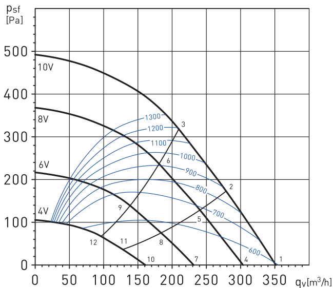
CAB-125 ECOWATT
