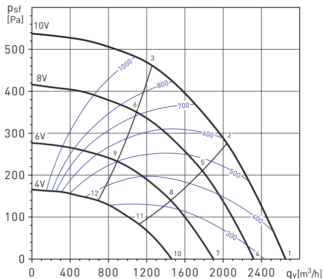
CAB-400 ECOWATT
