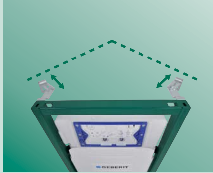
Geschikt voor hoekopstelling
