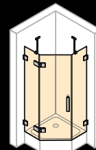
Zwaaideur met vaste segmenten, 1 vleu
