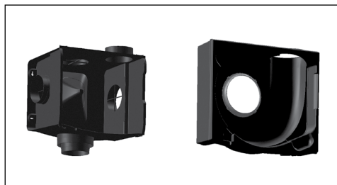
Fig. 14 Aanzuigplenum met slakkenhuis en inlaatrieg
