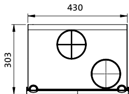
Fig. 3 Bovenaanzicht MVS-15R
